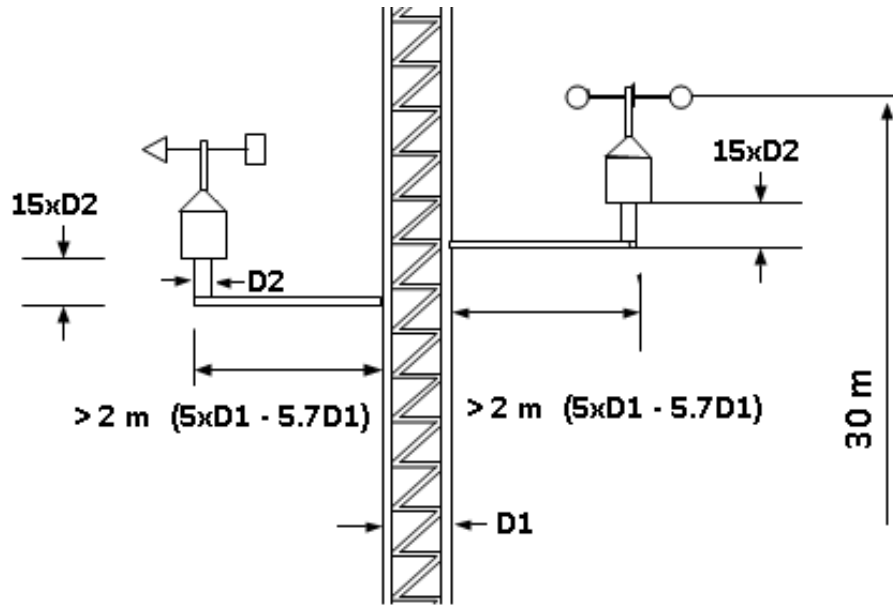
Şekil-4 : 30 m. Yükseklikte Rüzgar Ölçerler
