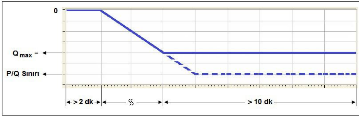
Şekil E.17.C.1.4 – Düşük İkazlı Reaktif Güç Desteği Testi Uygulanışı 58
