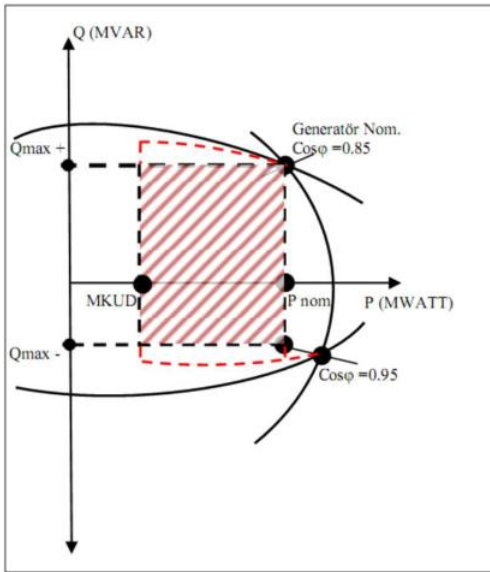
Şekil E.17.C.1.1 – Test Hedeflerinin Karşılandığı Durumlar (Jeneratör)
