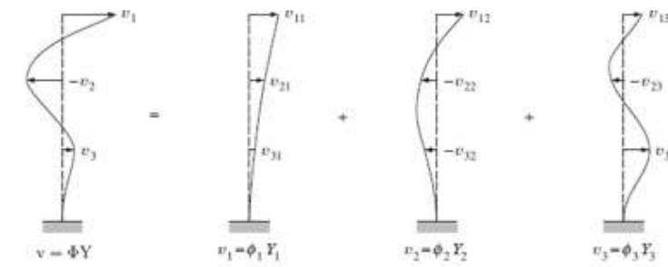
Şekil 3. Bir rüzgar türbini kulesinde görülecek titreşim mod şekilleri (soldan dağa: bileşke mod şekli, 1nci mod şekli, 2nci mod şekli, 3ncü mod şekli)
