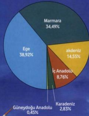
Kurulu gücün bölgelere göre dağılımı
